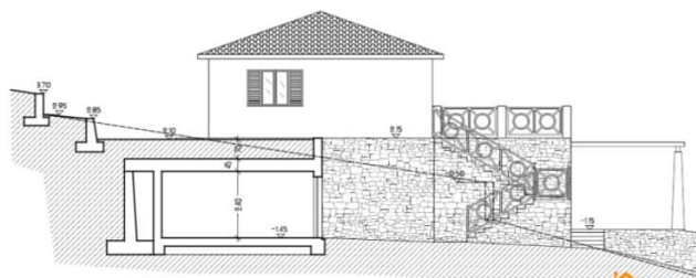
SEZIONE B-B
